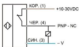
Тип выхода PNP - NC
