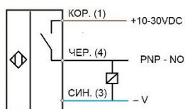
Тип выхода PNP - NO
