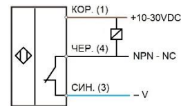
Тип выхода NPN - NC
