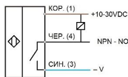
Тип выхода NPN - NO
